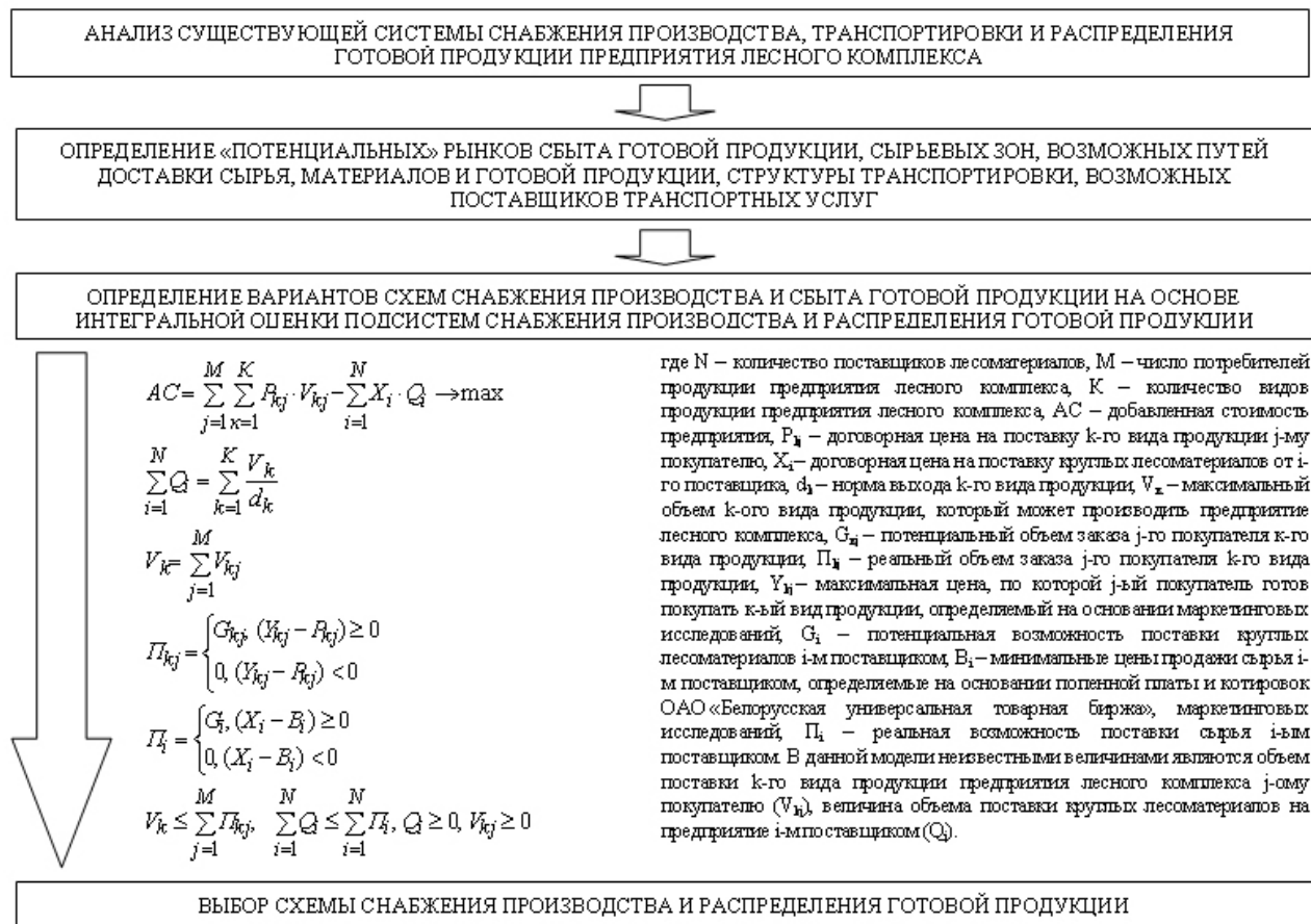
Рис. 4. Методика выбора рациональной схемы снабжения производства и распределения готовой продукции Fig. 4. Technique of a choice of the rational scheme of production supply and distribution of finished goods
