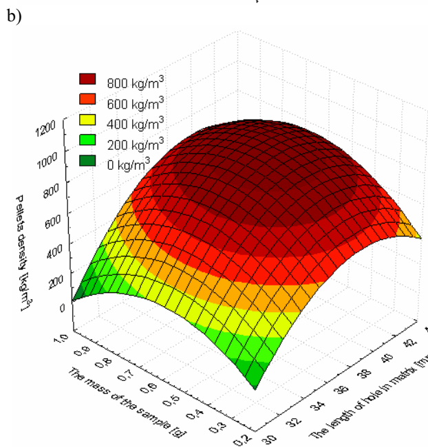
Fig. 2. The influence of material and process, and construction factors on the density of pellets obtained in the process of densification of a mixture of unshredded buckwheat hulls and potato pulp in an open chamber: a) the influence of potato pulp content and process temperature, b) the influence of the length of a matrix opening and the mass of the densified mixture Rys. 2. Wpływ czynników materiałowo-procesowych i konstrukcyjnych na maksymalne naciski zagęszczające uzyskane podczas zagęszczania mieszaniny nierozdrobnionej łuski gryki i wycierki ziemniaczanej w komorze otwartej: a) wpływ zawartości wycierki ziemniaczanej i temperatury procesu, b) długość otworu w matrycy i masa zagęszczanej próbki
