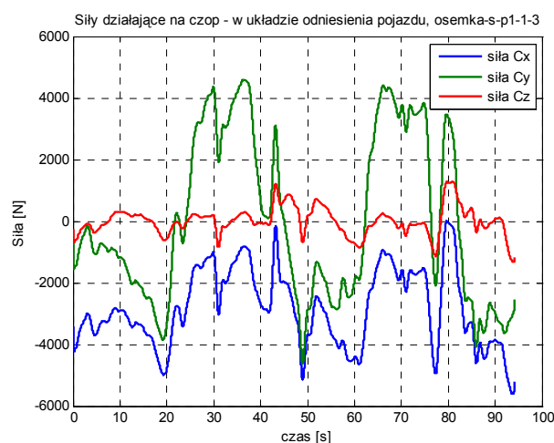
Rys. 8. Siły działające na czop zaczepu kulowego – w układzie odniesienia pojazdu Fig. 8. The forces acting on the hitch pin – reference system of the vehicle
