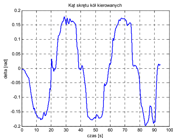
Rys. 7. Kąt skrętu kół przednich przy jeździe po torze ruchu w postaci "ósemki" Fig. 7. Steering angle of the front wheels – driving on the eight-shaped test track
