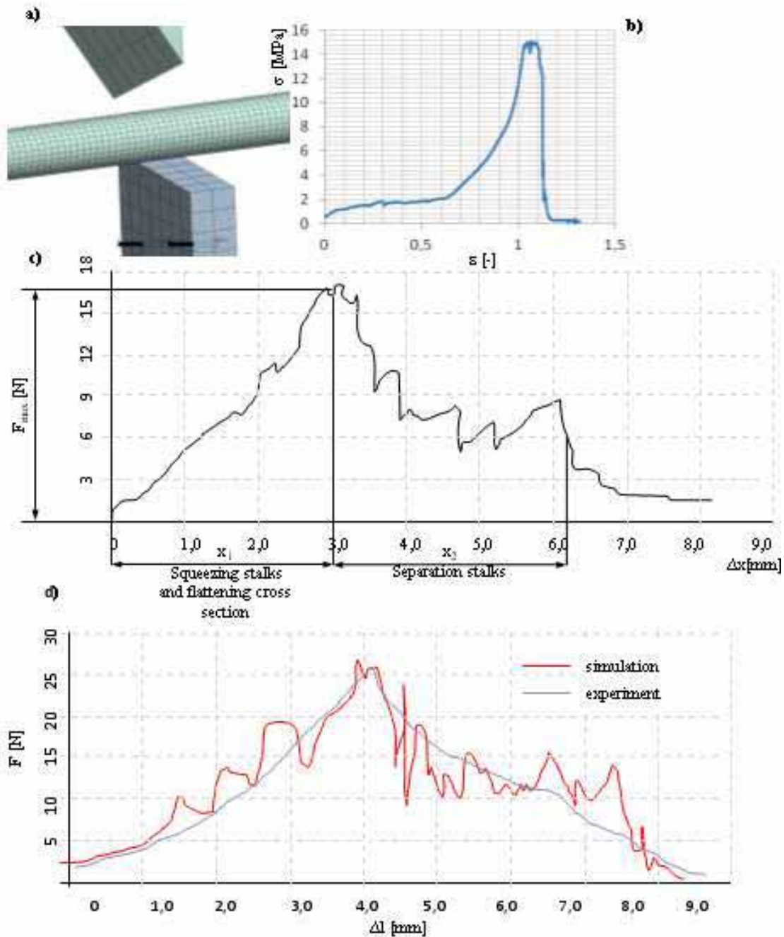
Fig. 4. View of the discrete numerical model (a), a graph \sigma = f(\epsilon) of the cutting stalks process, along with the phases [2] (c) cutting force change as a function of movement of the blade determined numerically and experimentally (d) Rys. 4. Widok dyskretnego modelu numerycznego (a), opracowany wykres \sigma = f(\epsilon) przebiegu procesu cięcia źdźbła, wraz z jego fazami [2] (c), zmiana sił cięcia w funkcji przemieszczenia noża wyznaczona numerycznie i eksperymentalnie (d)
