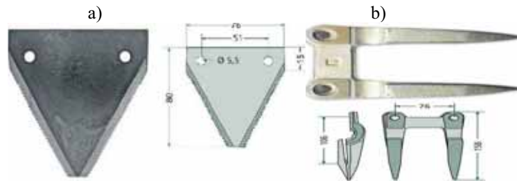
Fig. 5. Parts of the cutting assembly of harvester Bizon: a) knife, b) bayonet with finger liner [10, 11] Rys. 5. Części zespołu tnącego kombajnu Bizon: a) nóż, b) bagnet ze stalką [10, 11]
